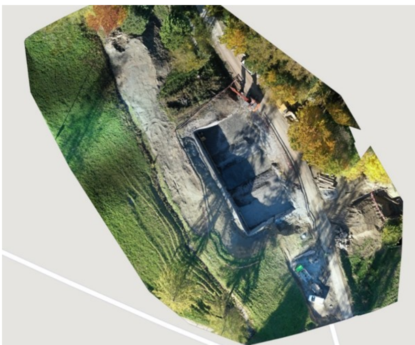
Figure 1 : Survol du chantier par drone en fin de terrassement
